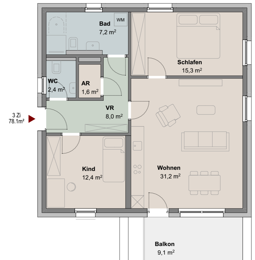
3 Zi 78.1m 2 2. OG
